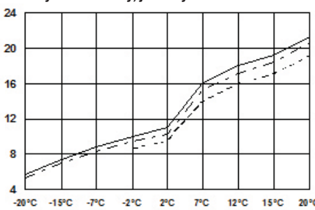
Výkonové křivky, jmen. výkon 14 kW - 3 fáze
