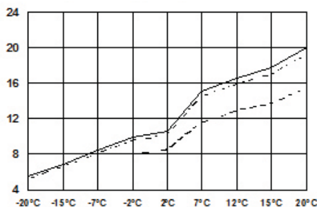
Výkonové křivky, jmen. výkon 14 kW - 3 fáze
