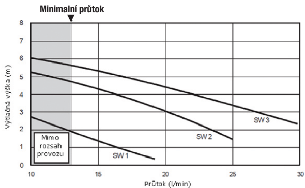
Charakteristika čerpadla HWS-803XWH (8kW)
