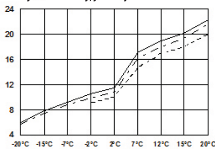
Výkonové křivky, jmen. výkon 16 kW - 3 fáze
