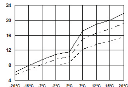
Výkonové křivky, jmen. výkon 16 kW - 3 fáze
