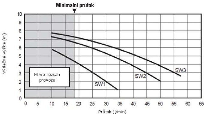
Charakteristika čerpadla HWS-1403XWH (11,14,16 kW)
