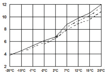
Výkonové křivky, jmen. výkon 11 kW - 3 fáze
